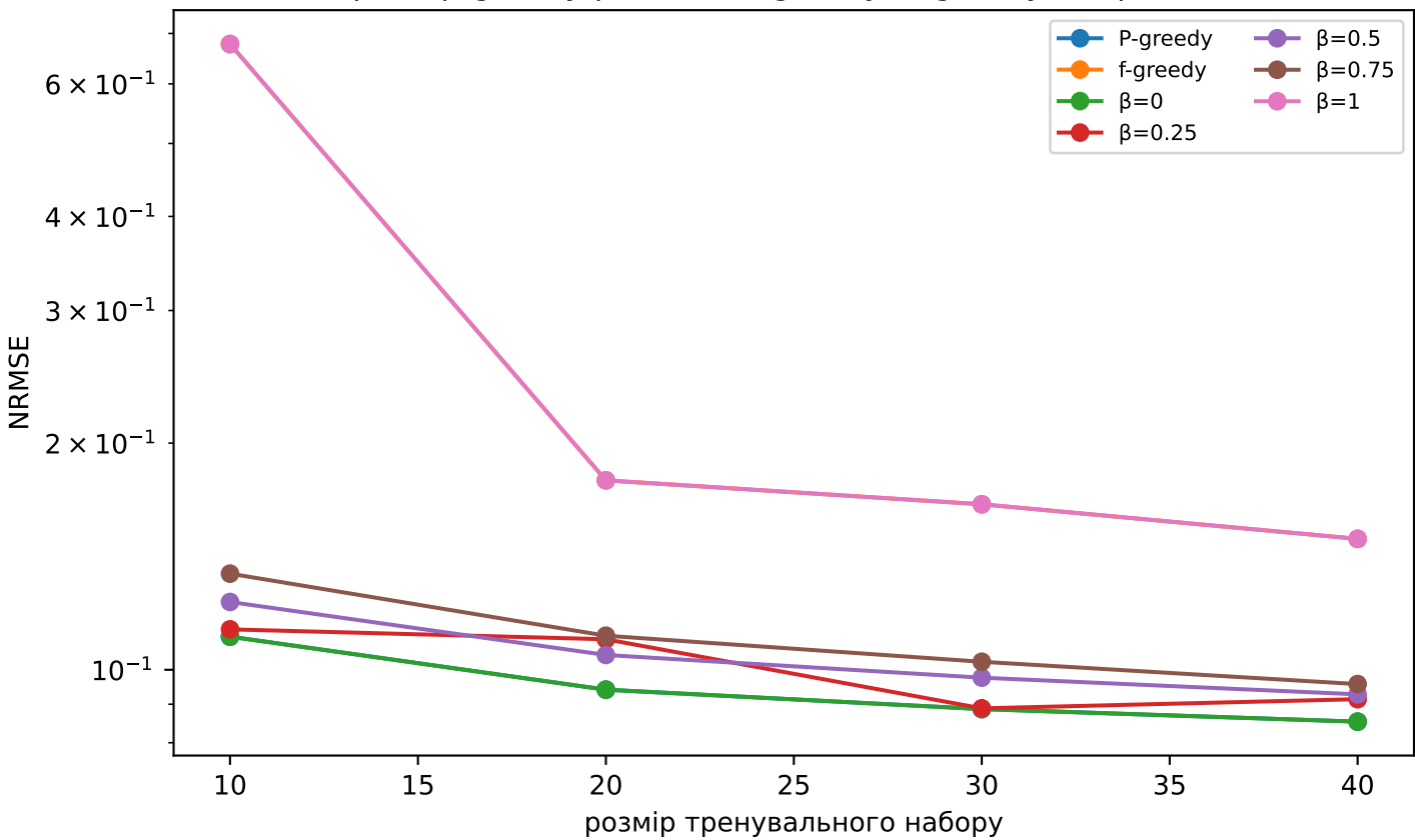
Розгортка \beta -greedy родини (P-greedy і f-greedy — крайні точки)
